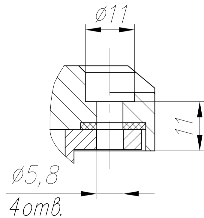
B-B(1:1)
